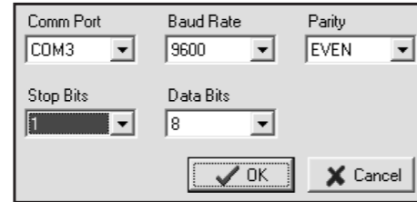
Janela definições (Parâm. Com) do programa BitBoy
