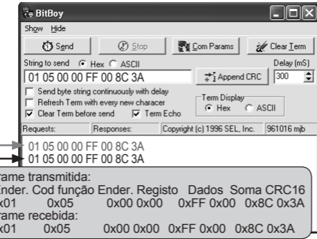
FC05 exemplo. Código transmissão pressionar botão 1.
