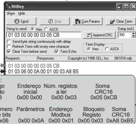
FC03 exemplo: Leitura registos.
